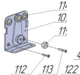
Рис.10.1 Закрепление при установке механизма на ЛЕВОМ щите корпуса
